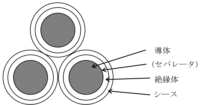
3心(FD-CVT)
