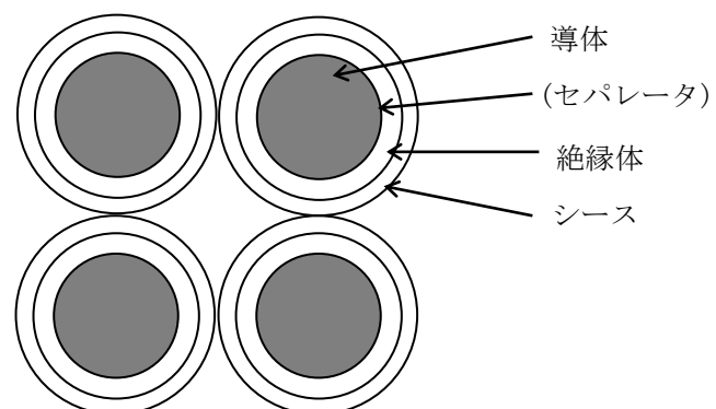
4心(FD-CVQ)
