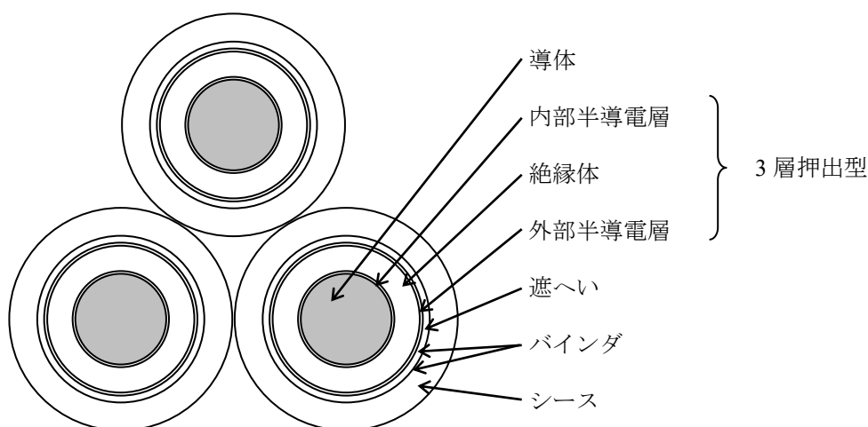
断面図
