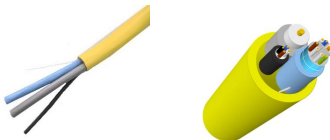
マルチメディア複合ケーブル「MLTT-10G1B11」
